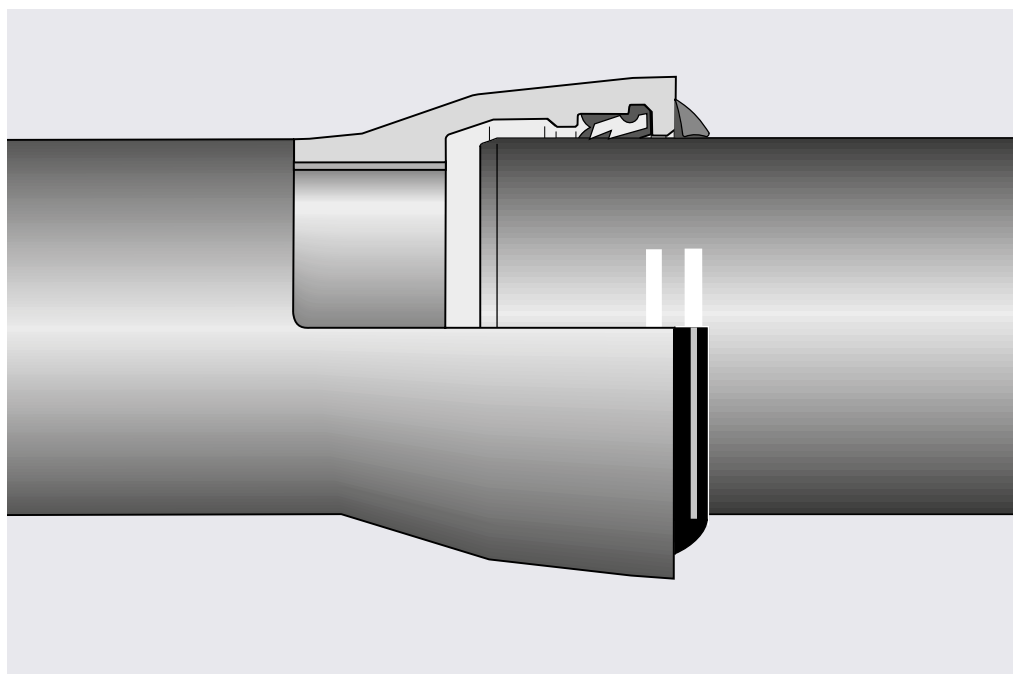
Längskraftschlüssige Muffenverbindung STANDARD Vi DN 80 - DN 700
