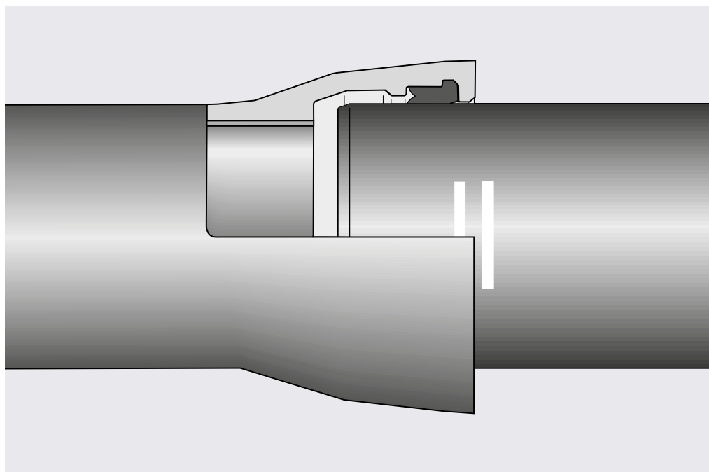
Steckmuffenverbindung STANDARD DIN 28603 DN 80 - DN 2000
