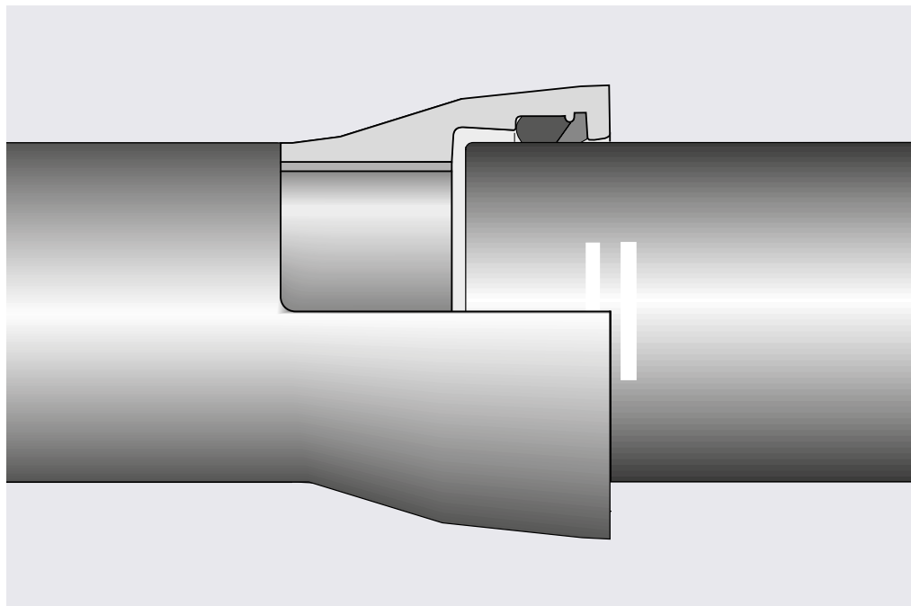
Steckmuffenverbindung TYTON DIN 28603 DN 80 - DN 300
