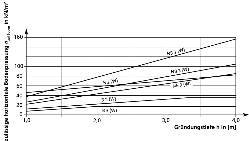
Diagramm 1: Zulässige horizontale Bodenpressung \sigma_{\text{zul.Boden}} in Abhängigkeit von Bodengruppe und Gründungstiefe h für Widerlager mit quadratischer Druckfläche ( h_G/b_G=1 ) unter Wasser
