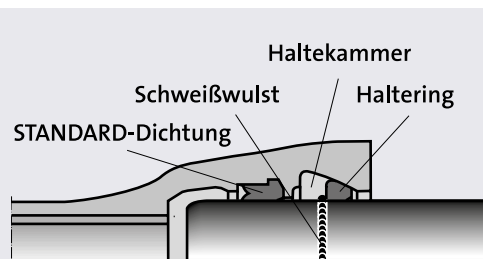
UNIVERSAL TIS-K mit STANDARD-Dichtung
