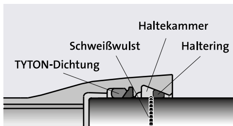
UNIVERSAL TIS-K mit TYTON - Dichtung
