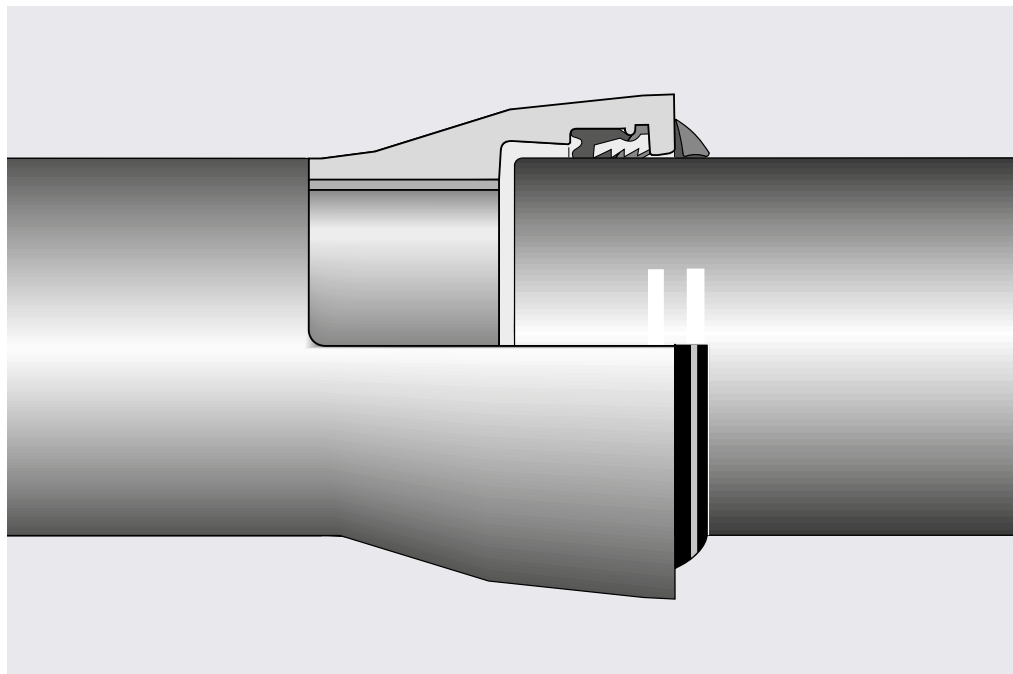
Längskraftschlüssige Muffenverbindung TYTON-SIT PLUS DN 80 - DN 300
