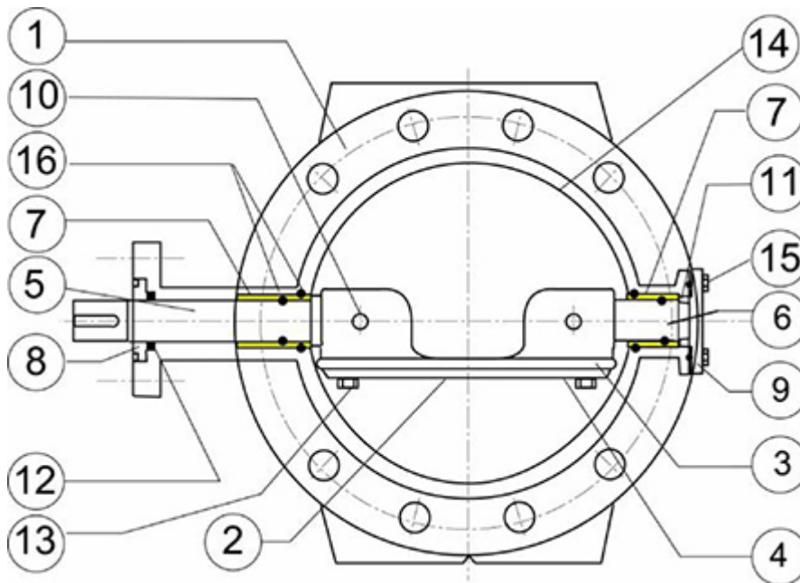
Ausführung DN900-2000 PN10 - DN800-2000 PN16 - DN700-2000 PN25
