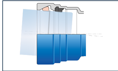
Kit ALPINAL Formstücke Universal Standard PECB + Verbindung Universal Standard TIS-K
