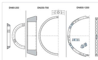
Haltering für Standard Ve Verbindung
