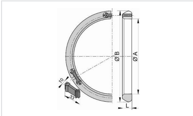
Haltering TIS-K
