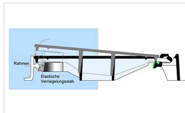
Schachtabdeckungen - Verschluss des Deckels mittels elastischen Verriegelungsstabs
