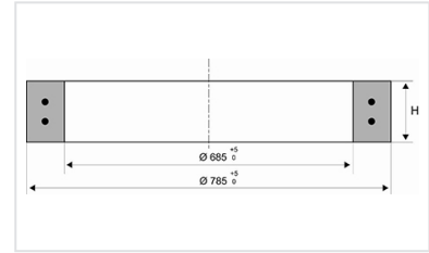
Beton-Adapterring - Schachtabdeckungen VIATOP NIVEAU
