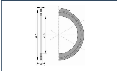
Flansch Dichtung für Flanschverbindung für ALPINAL
