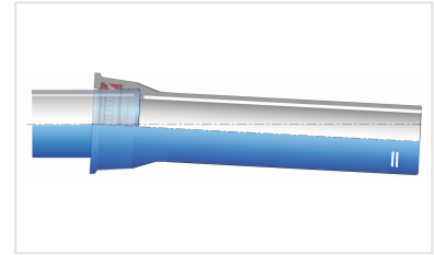
Kit Tyton Rohr + Tyton Sit- Plus Verbindung
