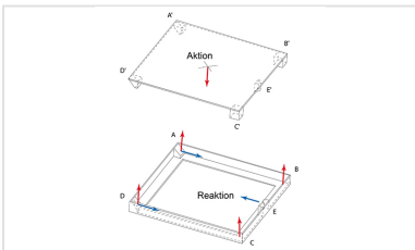
Schachtabdeckungen AKSESS Stabilität des Deckels
