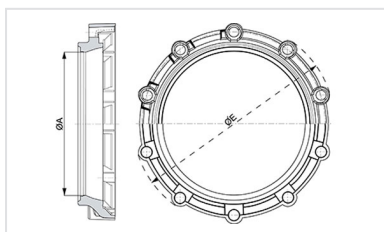
Contrabrida para Junta Standard Ve DN80-1200
