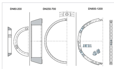
Anillo metálico para Junta Standard Ve DN80-1200
