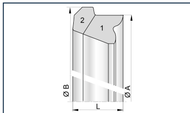
Junta de elastómero STANDARD HP para Tubería UNIVERSAL STANDARD C100, C64, C50
