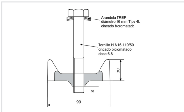
Elemento de encadenado para rejilla TRANSLINEA Clase D400 y E600
