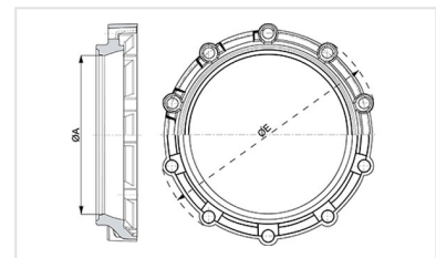
Contre-bride pour Joint STD Ve DN80-1200 (et joint STD V+i DN350-600)
