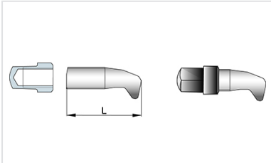
Boulon en fonte pour Joint STD Ve
