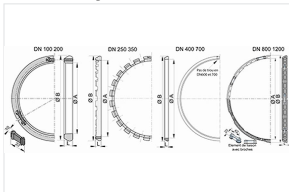
Joncs de verrouillage Standard Universal
