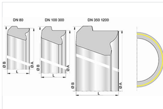
Rondelle Standard
