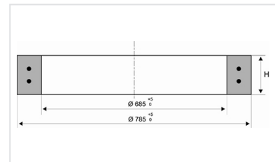
Bague béton pour Regards VIATOP 600 NIVEAU
