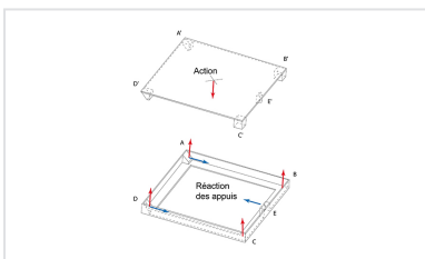
Info produit - Regards Hydrauliques AKSESS - Stabilité des tampons
