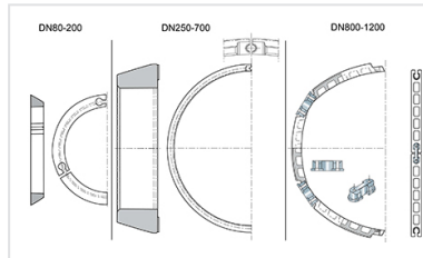
Jonc pour Joint STD Ve DN80-1200
