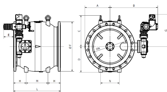
Version motorisée
