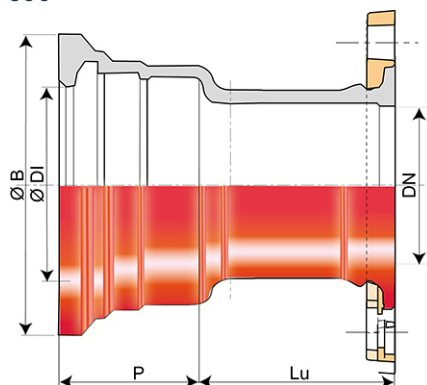
DN80-300
