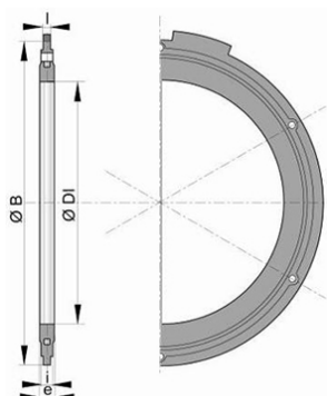
Gasket DN50-300 NBR
