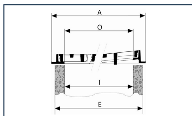
Grating SQUADRA C250 - Implementation
