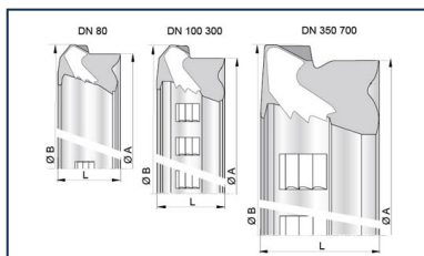
Gasket ViLoK® (NBR STD Vi) DN80-700
