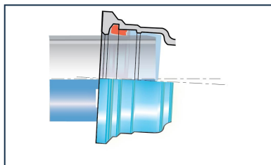
Conjunto Tê 2 bocas Standard/ flange PECB + Junta Standard
