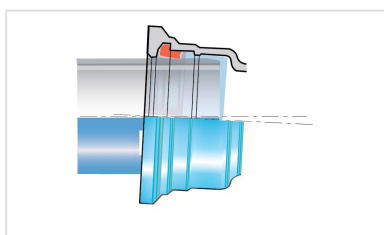
Conjunto cone bocas Standard AQB + Junta Standard
