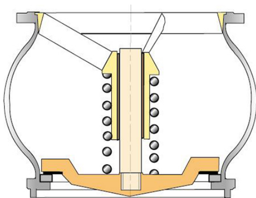
Válvula de retenção fechada
