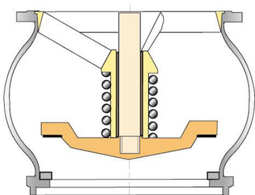
Válvula de retenção aberta
