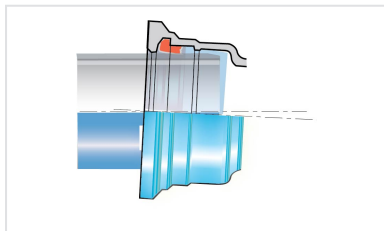
Conjunto curva Standard PECB + Junta Standard
