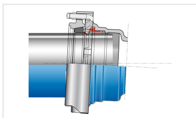
Conjunto acessório Standard PECEB + Junta Standard Ve
