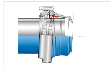
Conjunto acessório Standard PECEB + Junta Standard V+i
