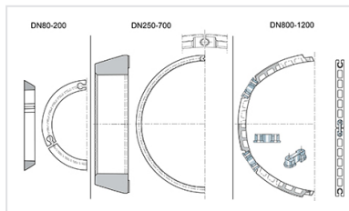
Anel travamento para STD Ve junta DN80-1200
