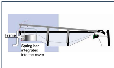
Tampas - Travamento por barra elástica
