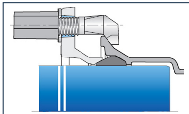
Conjunto para acessórios PECB Express + Junta Express
