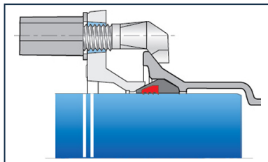
Conjunto acessório Express PECB + Junta Express Vi
