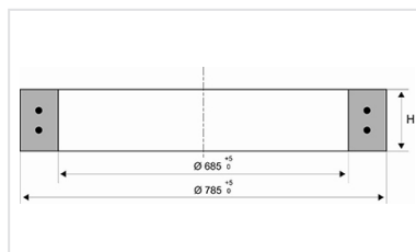
Beton-Adapterring - Schachtabdeckungen VIATOP NIVEAU
