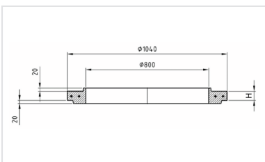
Auflagering VIATOP / PAMREX 800
