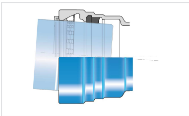
Kit Formstücke Universal Standard PCB + Verbindung Universal Standard NOVO-SIT
