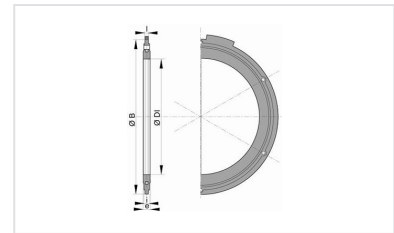
Flanschverbindung (galvanisiert) für Abwasser
