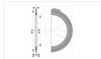
Flanschdichtungssatz (galvanisiert)
