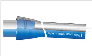
Kit Universal Tyton Rohr + Universal Tyton NOVO-Sit Verbindung
