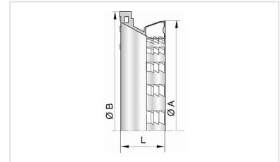
NOVO-SIT Haltering DN80-700
