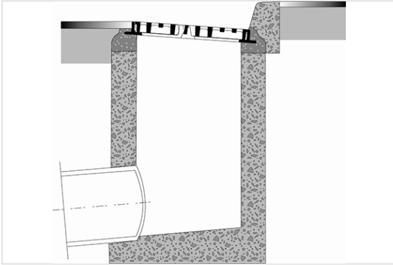
Ejemplo de instalación en un bordillo
