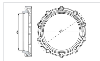
Contrabrida para Junta Standard Ve DN80-1200
