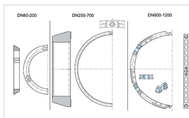
Anillo metálico para Junta Standard Ve DN80-1200
