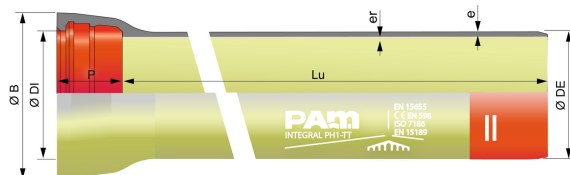
Tubería sin collerette DN150-1000
