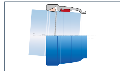
Kit Accesorio ALPINAL Universal Tyton PCB + Junta Universal Tyton Ve
