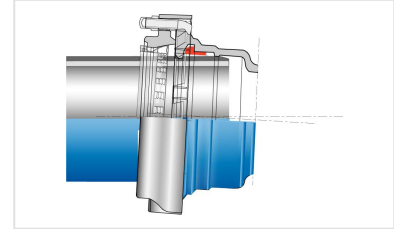
Kit Accesorio Standard PECB + Junta Standard V+i
