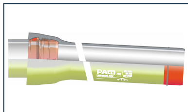
Kit Tubería Universal Standard Ve PUX + Junta Universal Standard Ve
