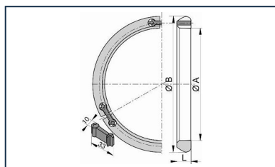
Junta de acerojado Universal Ve DN80-1800
