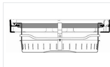
Seau à boue - Regards VIATOP
