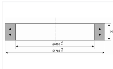
Bague béton pour Regards VIATOP 600 NIVEAU
