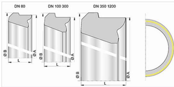
Rondelle Standard
