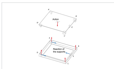
Tampa hidráulicas AKSESS - Estabilidade da tampa
