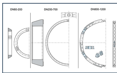
Anel travamento para STD Ve junta DN80-1200
