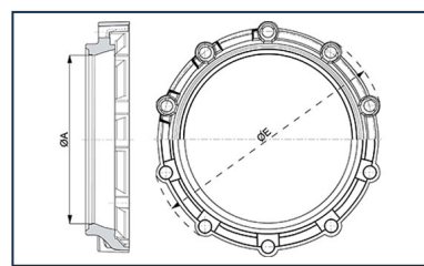
Contraflange STD Ve para junta DN80-1200
