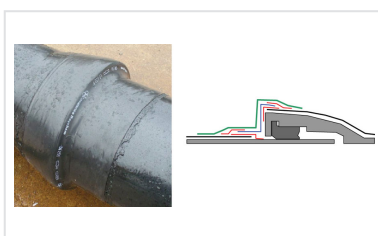
Instalação de manga de alumínio em tubos TT
