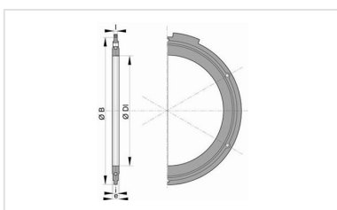
Conjunto de junta flangeada com parafusaria em aço galvanizado a quente
