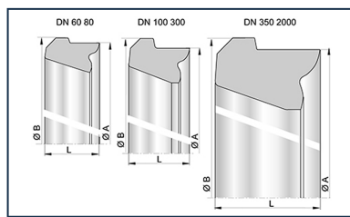
Junta Standard Junta para Tubos e acessórios DN60-2000
